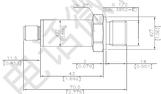
连接器 M12x1
