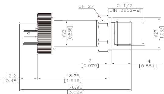
连接器EN 175301-803 C样式
