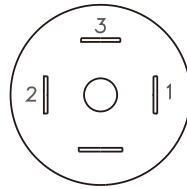
E-EN 175301-803
