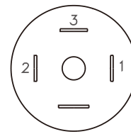
C-EN 175301-803
